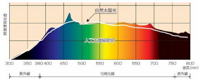
■人工太陽照明灯及び自然太陽光の分光分布
